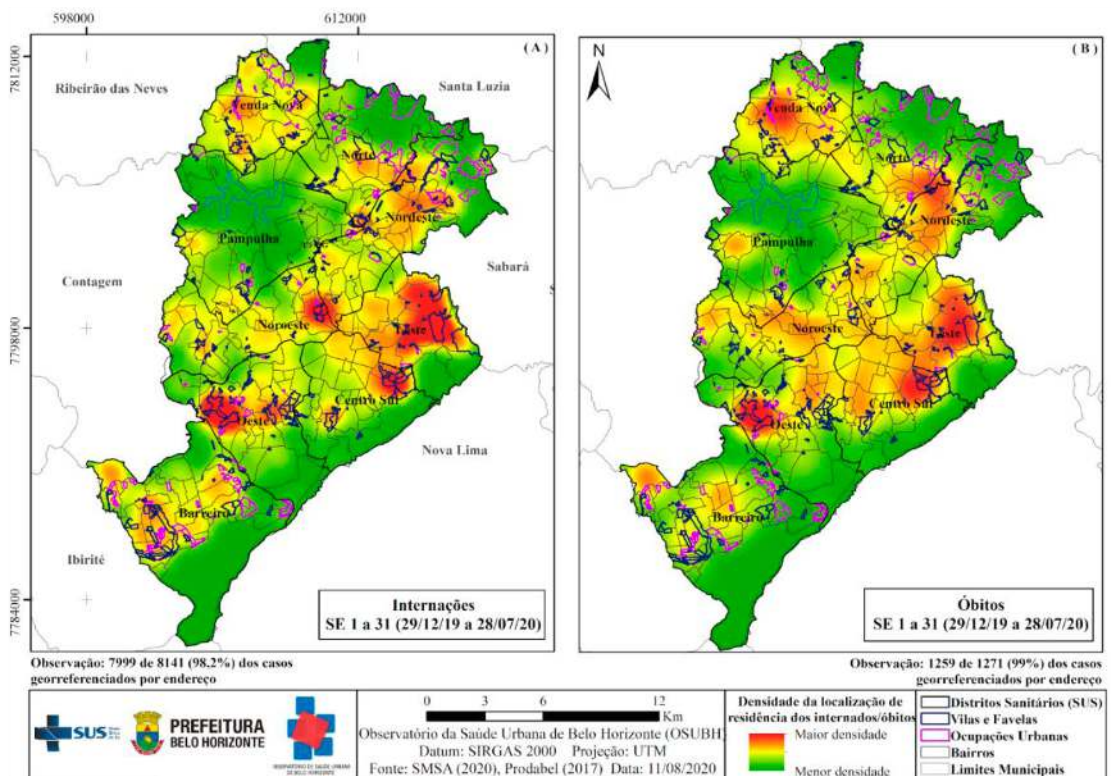
Figura 6: Comparação do resultado do experimento com Internações e óbitos da SE 1 a SE 31 (28/07/20). Fonte: InfoCOVID-OSUBH 6 (Sales et al., 18 August, 2020)
